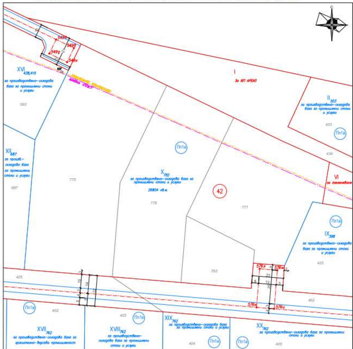
ПЛАН ЗА РЕГУЛАЦИЯ М 1:1000
